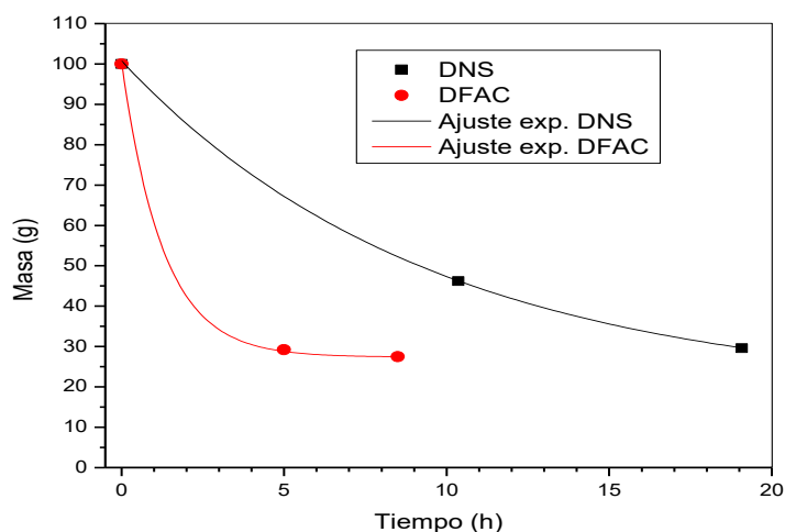
Figura 1. Comparativo del porcentaje de masa perdida (Humedad) por unidad de tiempo, entre las dos técnicas utilizadas, (DFAC y DNS).
